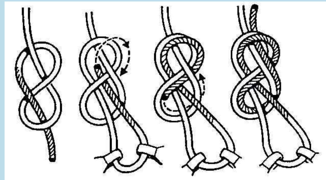
Nœud d'encordement en 8
